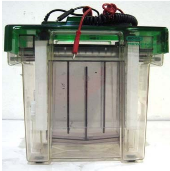
第二維：垂直電泳槽（2片裝） 型號: BioRad PII Xi Cell 應用: 主要用於SDS-PAGE分離用。
